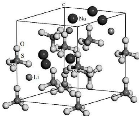
Рисунок 1. Кристаллическая структура \text{LiNaSO}_4 при комнатной температуре.
