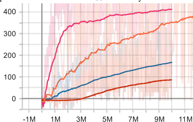
Рисунок 3. Очки игры за эпизод в зависимости от времени при разных алгоритмах
