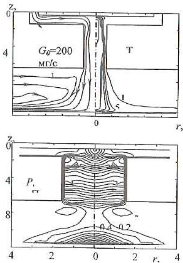
1-сүрөт. Газдын ток сызыктары ( G/G_0 = 0.05, 0.3, 0.9, 1.5, 2, 2.5 ), изотермалар ( T = 1, 5, 8, 10, 12, 15 kK) жана басым талаасы (кадам 0.2 kПа); I = 70A .
