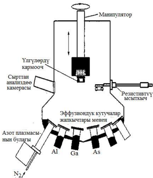
1 - сүрөт. \text{Al}_x\text{Ga}_{1-x}\text{As} – GaAs гетероструктурасын молекулярдык – нур эпитаксия ыкмасы менен өстүрүү
