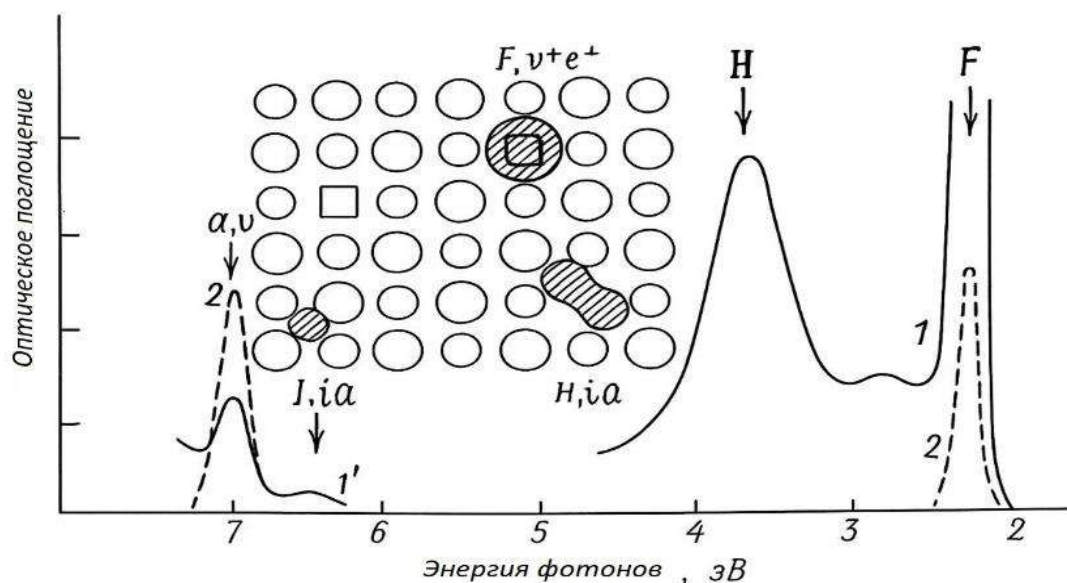
Рисунок 6. Центры окраски и спектры оптического поглощения в щелочно-галогидных кристаллах.
