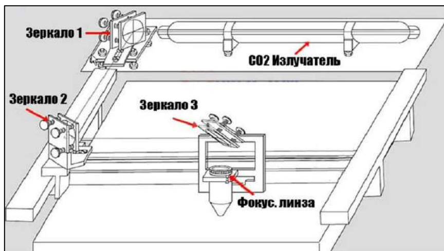
1-сүрөт. CO 2 -лазери менен орнотмонун схемасы.
