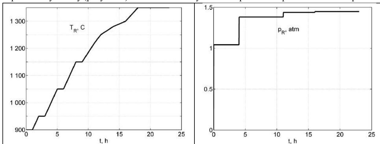
Рисунок 1. Зависимость температуры и давления азота в печи в условиях реакционного спекания изделий в лаборатории порошковых материалов ИФ им. Ж.Жээнбаева НАН КР [4].
