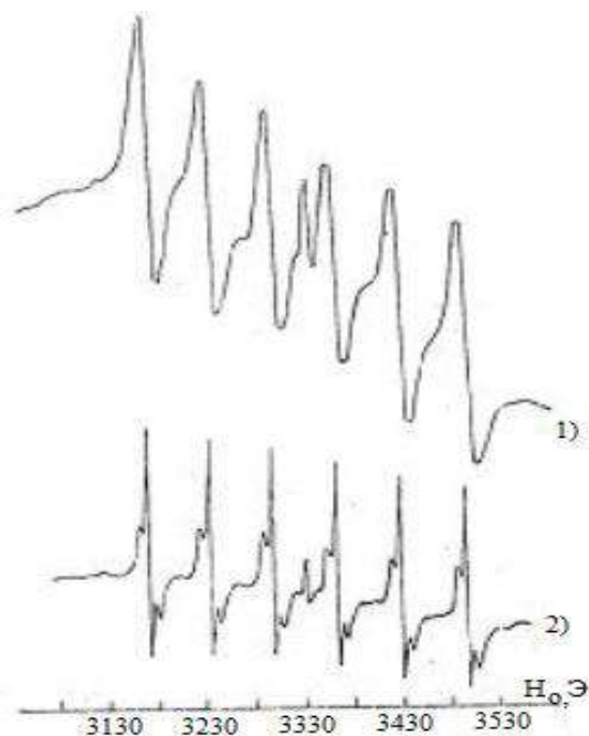
4-сүрөт. \text{Pb}_{1-x}\text{Ge}_x\text{Te:Mn}(x=0,03) монокристаллдарынын T = 20\text{ K} температурадагы (а – 5 саат нурдантуудан кийин, б) – 10 саат нурдантуудан кийин, W = 25\text{ Вт/см}^2 жазылып алынган ЭПР спектрлери.
