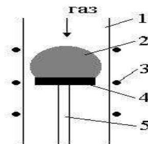
3 - сүрөт. Разрядды электродсуз жогорку жыштыкта кызытып жана кармап туруучу тутумдун схемасы:
