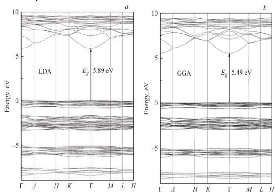
Рисунок 2. Рассчитанная зонно-энергетическая диаграмма для кристалла \text{LiNaSO}_4 с использованием функционалов LDA (a) и GGA (b)
