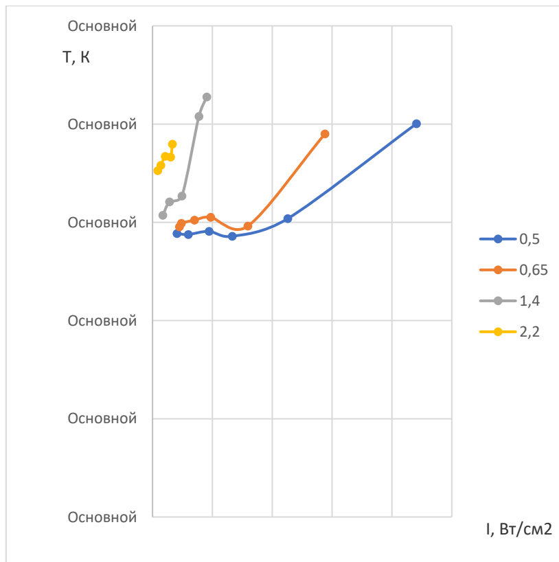
Рис. 3. Экспериментальные зависимости T(I) при различных d .
