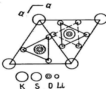
Рисунок 3. Проекция элементарной ячейки на плоскость "aa", пунктирный треугольник соответствует фазе P31c
