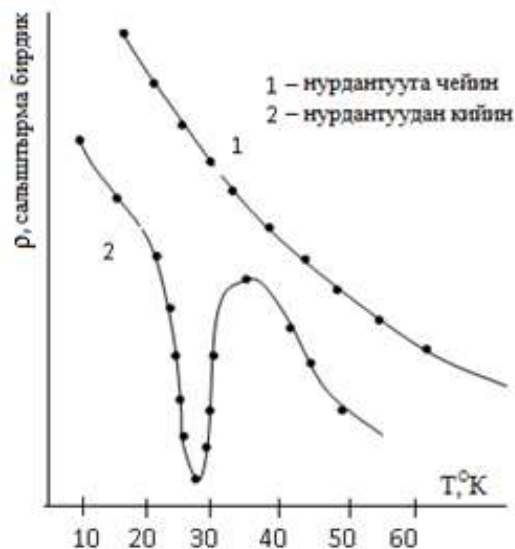
2-сүрөт. \text{Pb}_{1-x}\text{Ge}_x\text{Te:Mn} ( x = 0,03 ) жарым өткөргүчүнүн салыштырма электрдик каршылыгынын \rho(T) температуранын 4,2^\circ\text{K} < T < 30^\circ\text{K} аймагында көз карандылыгы.
