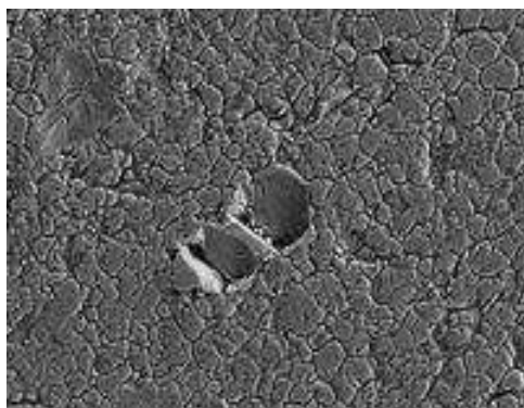
Рисунок 5.а) Поры, б)Включения
