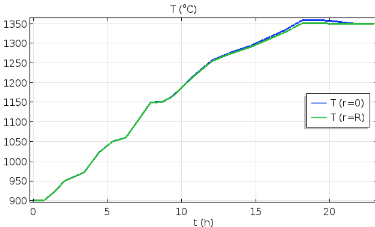
Рисунок 2. Эволюция температуры на оси и поверхности цилиндрического изделия: максимальный перепад температуры ( \sim 10 °C) наблюдается в момент времени t = 18,3 ч.
