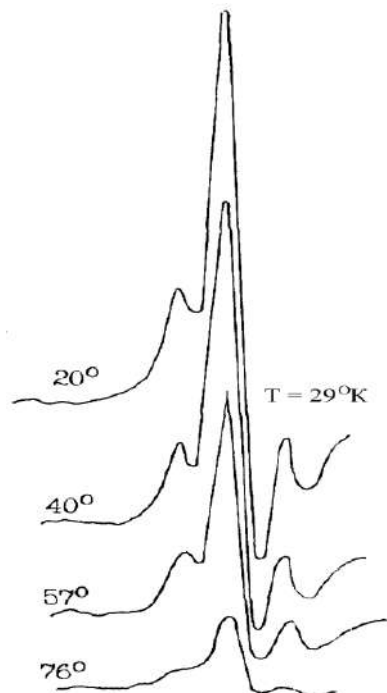
5-сүрөт. \text{Pb}_{1-x}\text{Ge}_x\text{Te:Mn} ( x=0,03 ) монокристаллынын ЭПР сызыктарындагы T = 29\text{ K} температурада бурчтук көз карандылыктары.
