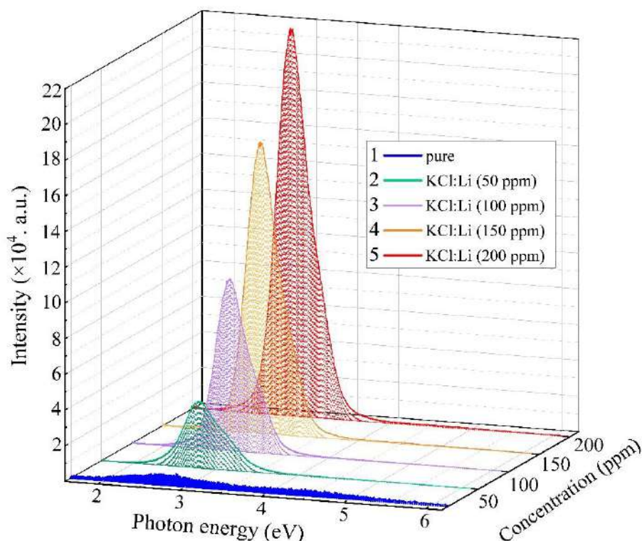
Рисунок 3. Спектры рентгенолюминесценции кристаллов при 300К: 1 – KCl (чистый), 2 – KCl:Li (50 ppm), 3 – KCl:Li (100 ppm), 4 – KCl:Li (150 ppm), 5 – KCl:Li (200 ppm).
