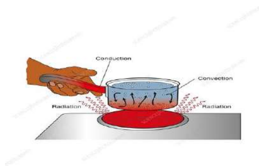
5-сүрөт. Конвекция
