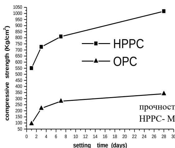
Рис. 3: Результаты портландцемент,
