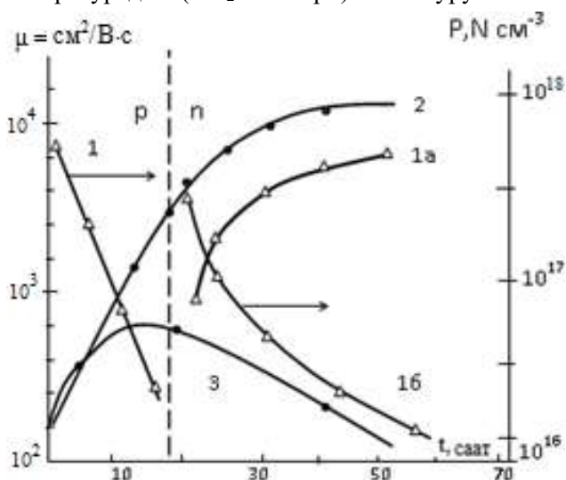
1-сүрөт. PbTe:Mn , Pb_{1-x}Ge_xTe:Mn ( x= 0,03 ) жарым өткөргүчтөрүнүн заряд ташуучуларынын концентрациясынын ( p , n ), кыймылдуулугунун ( \mu ) лазер нуру менен нурдантуу убактысынан ( t ) көз карандылыгы.
