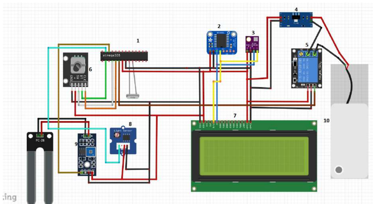
Рис.7. Принципиальная схема
