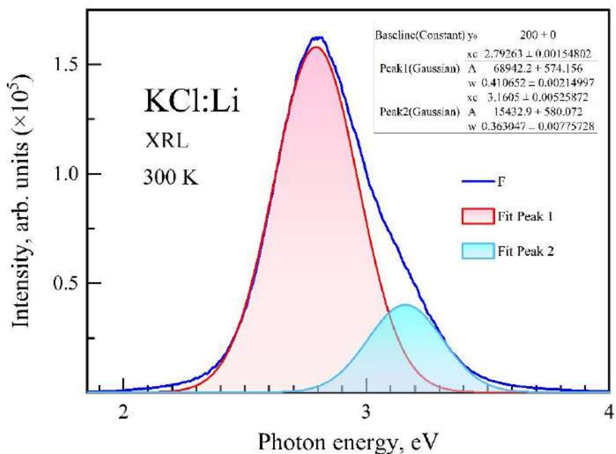
Рисунок 4. Спектр рентгенолюминесценции кристалла KCl:Li (150 ppm), разложенный на две гауссовы составляющие с максимумами при 2.8 эВ и 3.1 эВ. Регистрация спектров осуществлена при 300 К.
