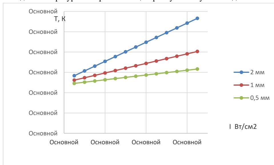
Рис. 4. Зависимость температуры зоны воздействия от интенсивности ЛИ при различных диаметрах лазерного пучка.
