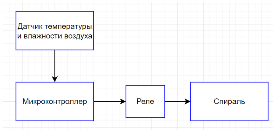
Рис.5. Структурная схема подогрев воздуха.
