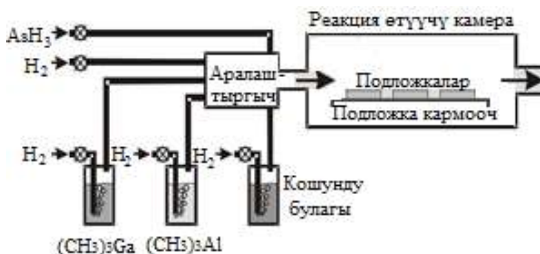
2 - сүрөт. МОБ – гидрид технологиясында GaAs - Al_xGa_{1-x}As суперкаптамдарын өстүрүү түзүмүнүн схематикалык сүрөттөлүшү
