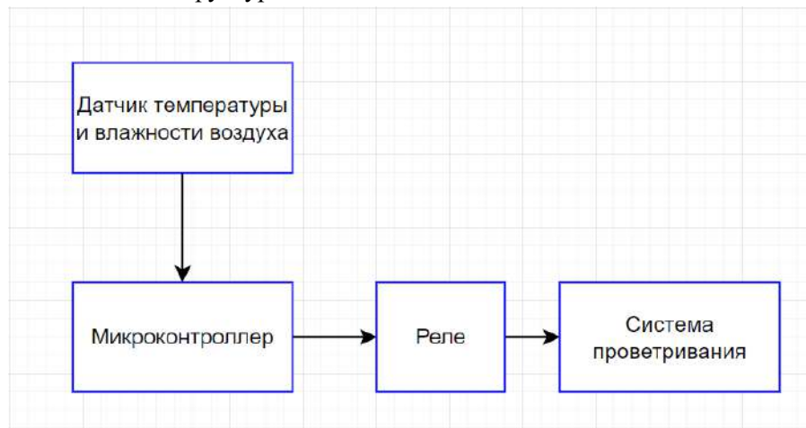
Рис.3. Структурная схема авто проветривания
