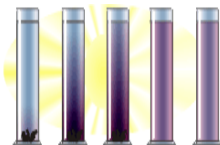
Рис. 3. Демонстрация процесса диффузии в жидкости
