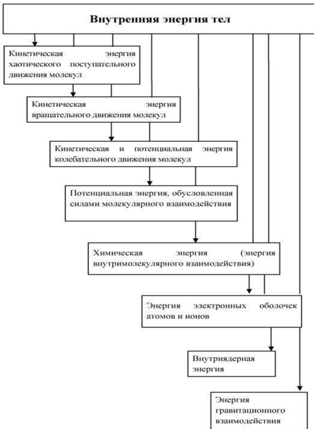
Рис. 1. Структура внутренней энергии вещества
