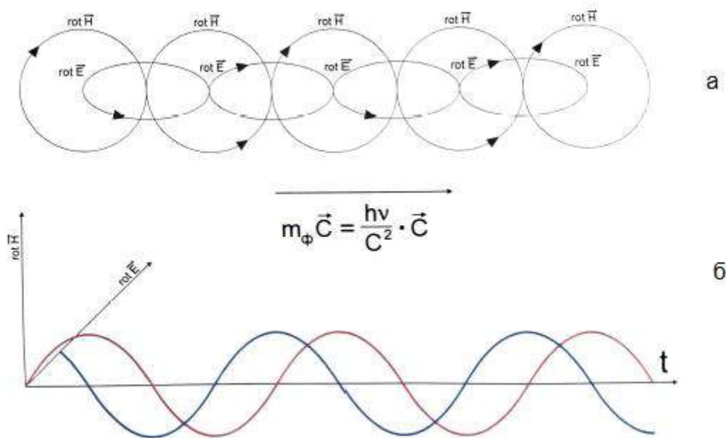
Рисунок 1. График электромагнитного излучения в пространстве.
