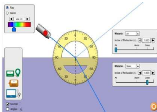
Сүрөт 1. Жарыктын сынуусун моделдөө
