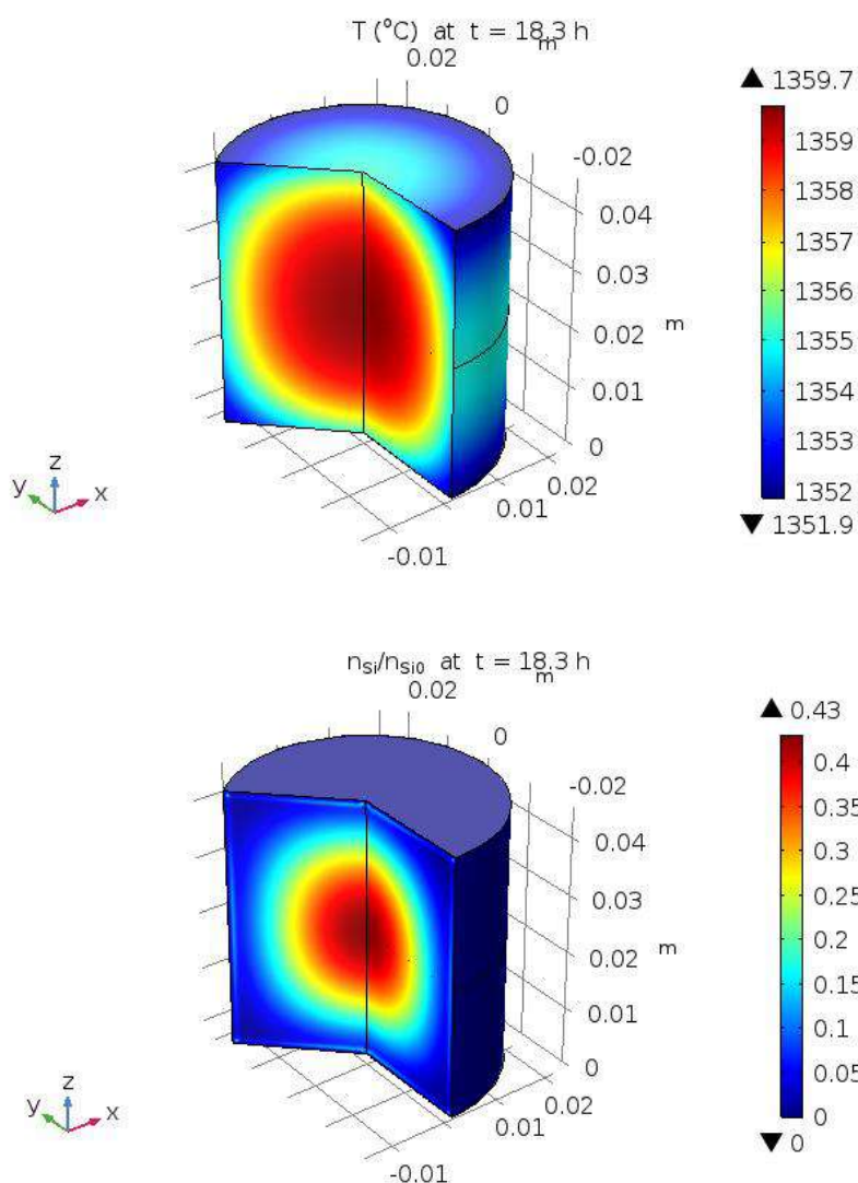
Рисунок 3. Пространственное распределение температуры и относительной концентрации атомов кремния в изделии в момент времени 18,3 ч после начала спекания.
