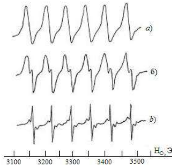
3-сүрөт. PbTe:Mn (2) монокристаллдарынын T = 20 К температурадагы: а) – 5 саат нурдантуудан кийин, б) – 10 саат нурдантуудан кийин, в) W = 25 Вт/см 2 жазылып алынган ЭПР спектрлери.
