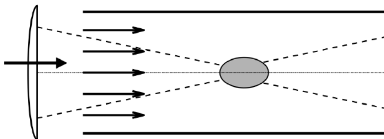
Рисунок 1. Схема непрерывного оптического разряда.
