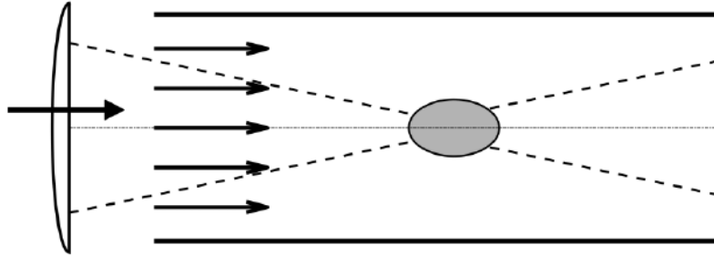
Рисунок 1. Схема непрерывного оптического разряда.
