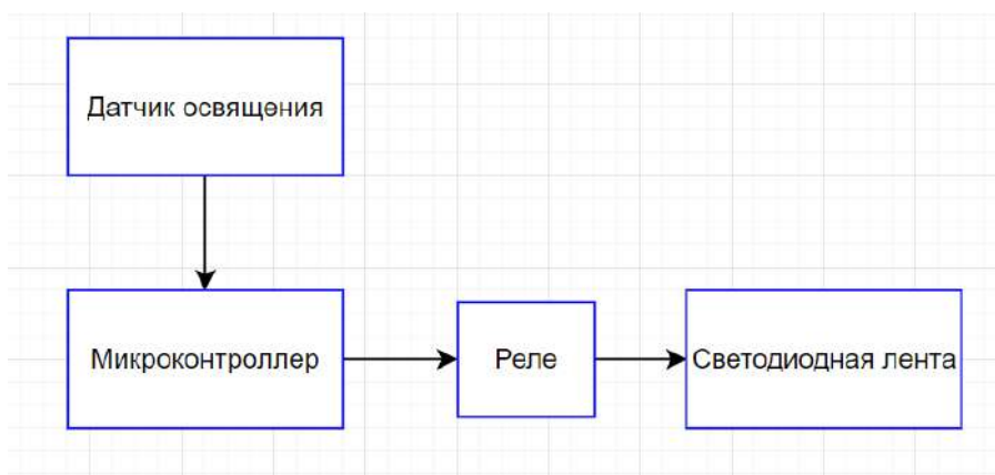
Рис.4. Структурная схема искусственного освещения
