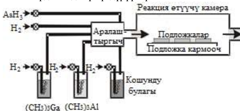
2 - сүрөт. МОБ – гидрид технологиясында \text{GaAs} - \text{Al}_x\text{Ga}_{1-x}\text{As} суперкаптамдарын өстүрүү түзүмүнүн схематикалык сүрөттөлүшү
