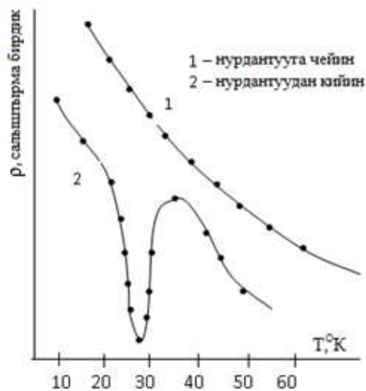
2-сүрөт. \text{Pb}_{1-x}\text{Ge}_x\text{Te:Mn} ( x = 0,03 ) жарым өткөргүчүнүн салыштырма электрдик каршылыгынын \rho(T) температуранын 4,2^\circ\text{К} < T < 30^\circ\text{К} аймагында көз карандылыгы.
