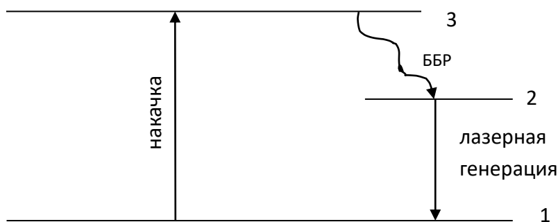
Рис.2. Трехуровневая схема накачки.
