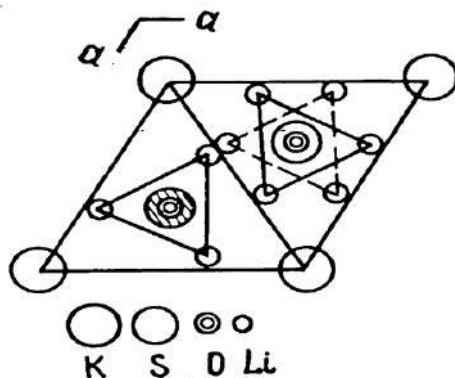
Рисунок 3. Проекция элементарной ячейки на плоскость "aa", пунктирный треугольник соответствует фазе P31c
