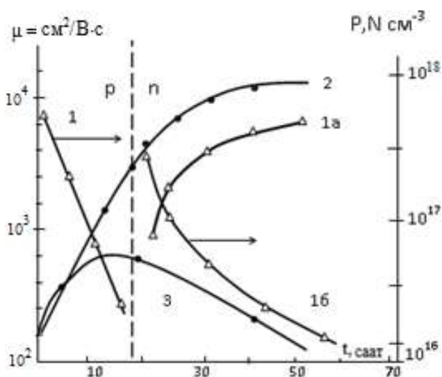
1-сүрөт. PbTe:Mn , Pb_{1-x}Ge_xTe:Mn ( x = 0,03 ) жарым өткөргүчтөрүнүн заряд ташуучуларынын концентрациясынын ( p , n ), кыймылдуулугунун ( \mu ) лазер нуру менен нурдантуу убактысынан ( t ) көз карандылыгы.
