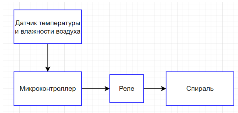
Рис.5.Структурная схема подогрев воздуха. Алгоритм работы устройства представлен на Рис.6.
