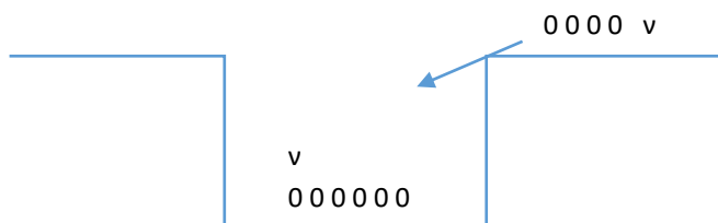
1–сүрөт. Потенциалдык чуңкурдан когерент энергия менен чыгуу
