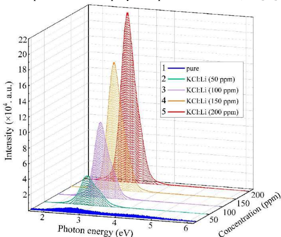
Рисунок 3. Спектры рентгенолюминесценции кристаллов при 300K: 1– KCl (чистый), 2 – KCl:Li (50 ppm), 3 – KCl:Li (100 ppm), 4 – KCl:Li (150 ppm), 5 – KCl:Li (200 ppm).
