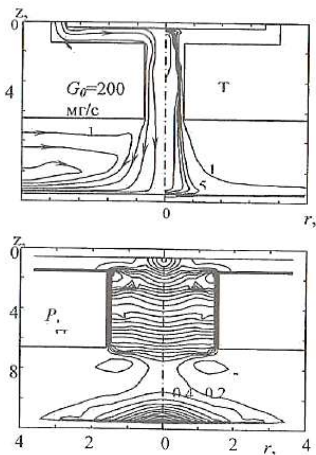
1-сүрөт. Газдын ток сызыктары ( G/G_0 = 0.05, 0.3, 0.9, 1.5, 2, 2.5 ), изотермалар ( T = 1, 5, 8, 10, 12, 15 kK) жана басым талаасы (кадам 0.2 kПа); I = 70 А.
