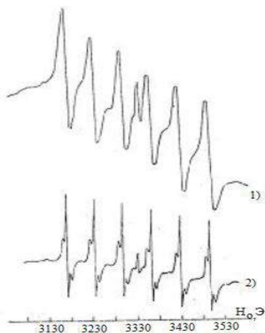
4-сүрөт. \text{Pb}_{1-x}\text{Ge}_x\text{Te:Mn}(x=0,03) монокристаллдарынын T = 20\text{ K} температурадагы (а – 5 саат нурдантуудан кийин, б) – 10 саат нурдантуудан кийин, W = 25\text{ Вт/см}^2 жазылып алынган ЭПР спектрлери.
