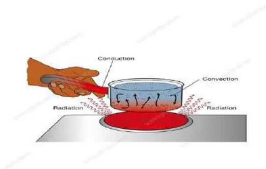
5-сүрөт. Конвекция
