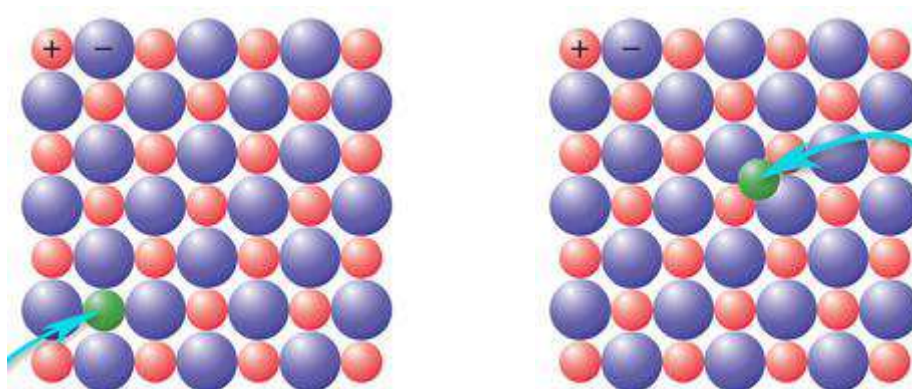
а)Примесь замещения
