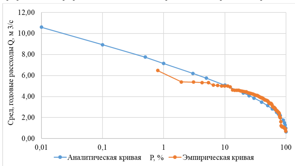
Рис. 4. Логарифмический график среднегодовых расходов воды
