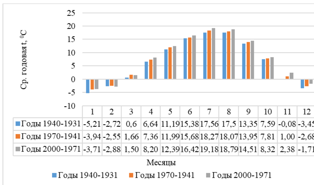
Рис. 2. Среднегодовая температура на м/с Рыбачье за период 1931-2000 годы
