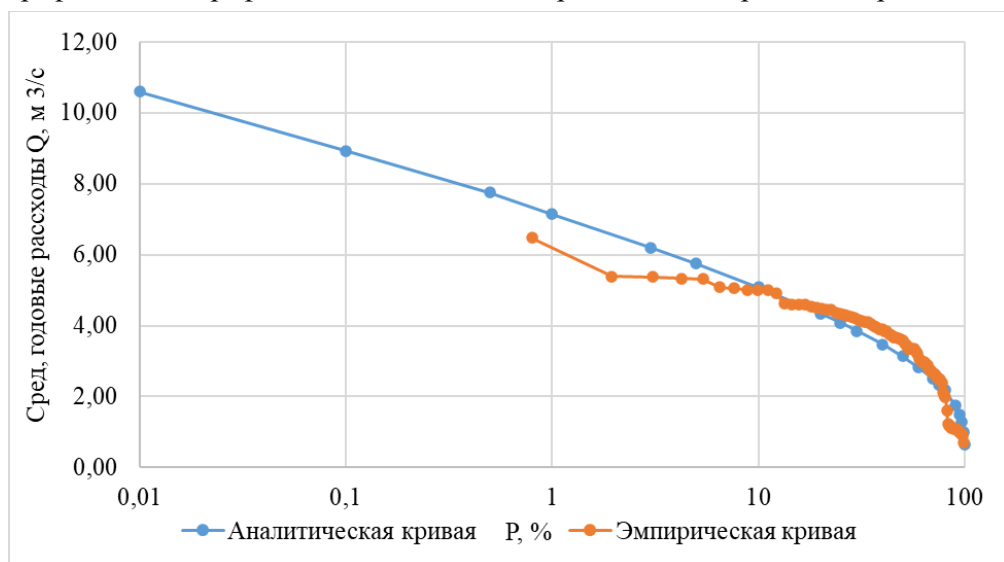
Рис. 4. Логарифмический график среднегодовых расходов воды
