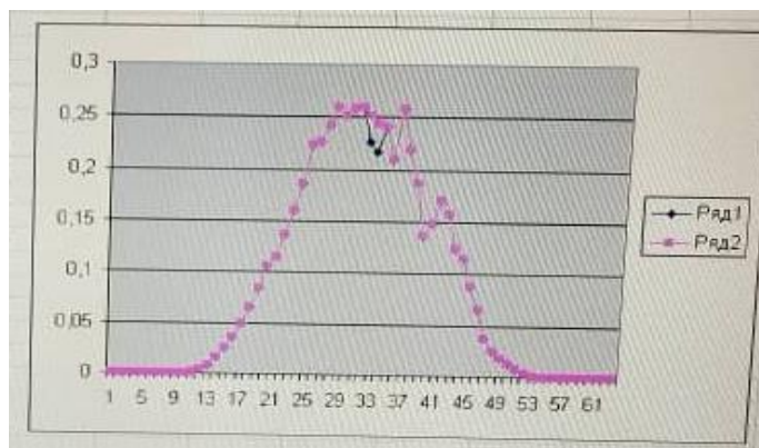
1-сүрөт. Ультракызылткөк нурунун 2025ж.февраль айындагы өзгөрүүсү: \text{W}/\text{м}^2 (\text{t})
