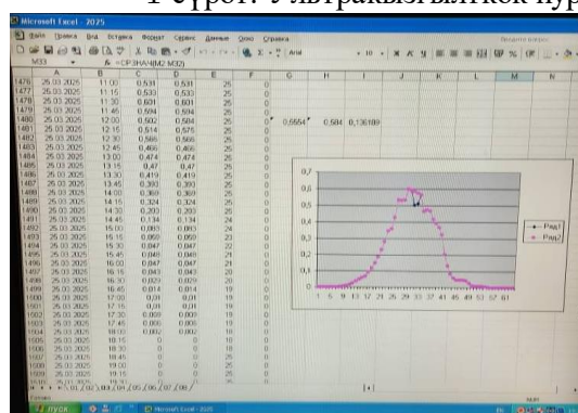
2-сүрөт. Ультракызылткөк нурунун 2025-ж.март айындагы өзгөрүүсү : \text{W}/\text{м}^2 (\text{t})
