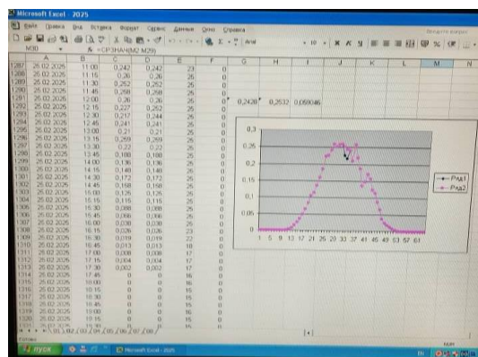
1-сүрөт. Ультракызылткөк нурунун 2025ж.февраль айындагы өзгөрүүсү: \text{W}/\text{м}^2 (\text{t})
