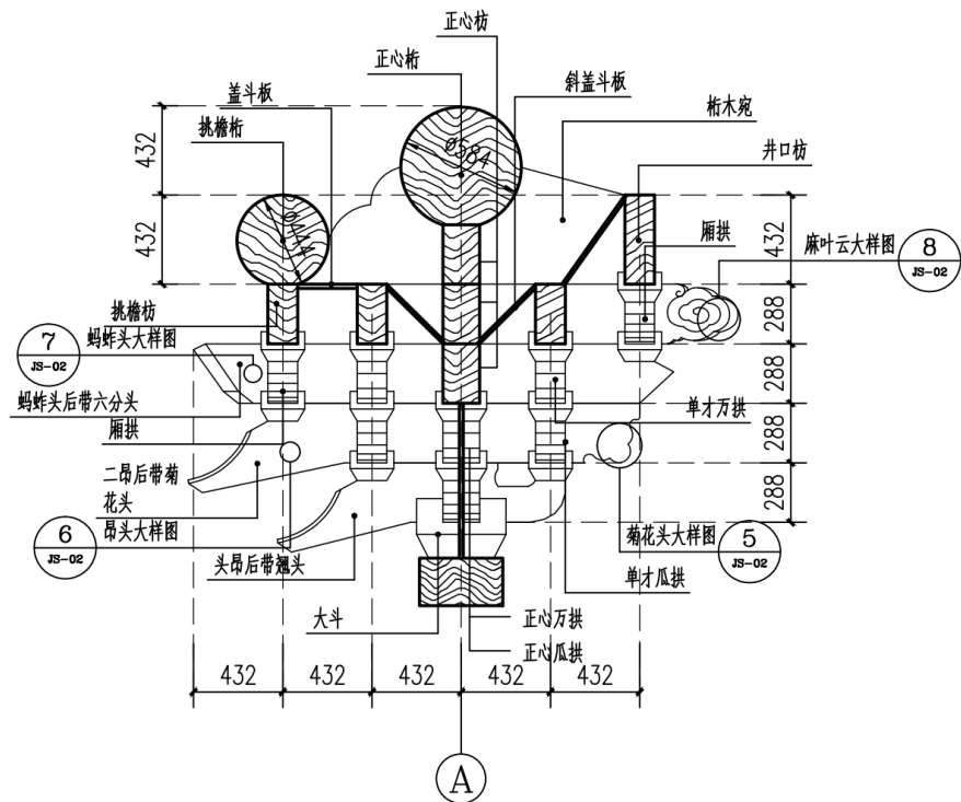
图 1 选用的四等材重昂五踩斗拱平身科侧立面图
