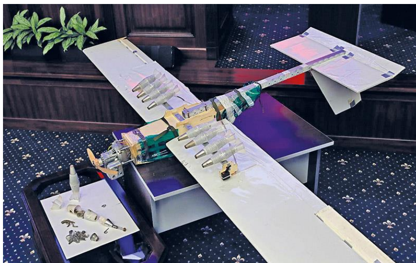
Рис. 1. Внешний вид БПЛА, перехваченных российскими подразделениями РЭБ в январе 2018 года
