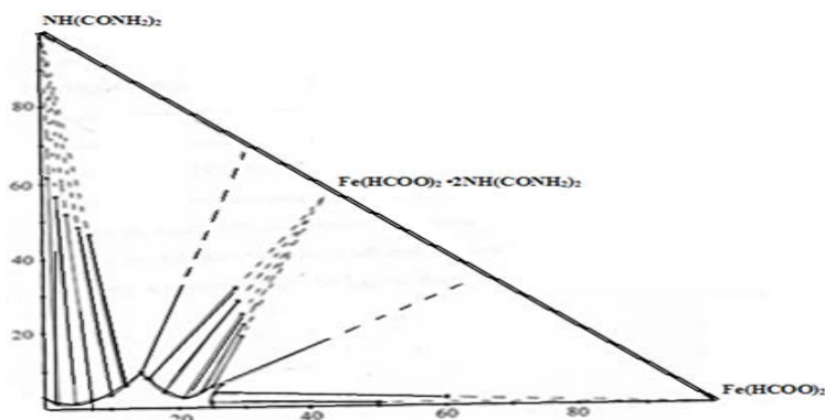
Рис.1 Диаграмма растворимости системы \text{Fe}(\text{HCOO})_2 - \text{NH}(\text{CONH}_2)_2 - \text{H}_2\text{O} при 25^\circ\text{C} .
