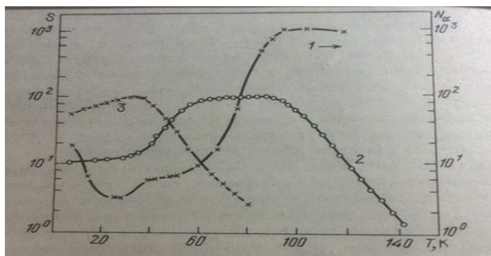
Рис.1. Температурные зависимости эффективности создания Х-облучением -центров в кристаллах КИ (1), а так же температурные зависимости люминесценции 3,3 эВ АЛЭ (2) и 5,83 эВ СЭ (3) при облучении КИ фотонами 6,02 ЭВ [6].
