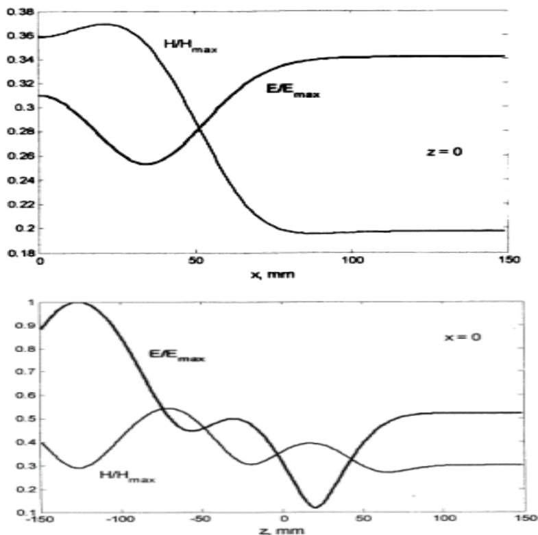
Рис.2. Распределение напряженностей электрического и магнитного полей вдоль осей x и z при ромбической камере: L_{camera} = 154 мм, E_{max} = 15 кВ/м, H_{max} = 34.44 А/м.
